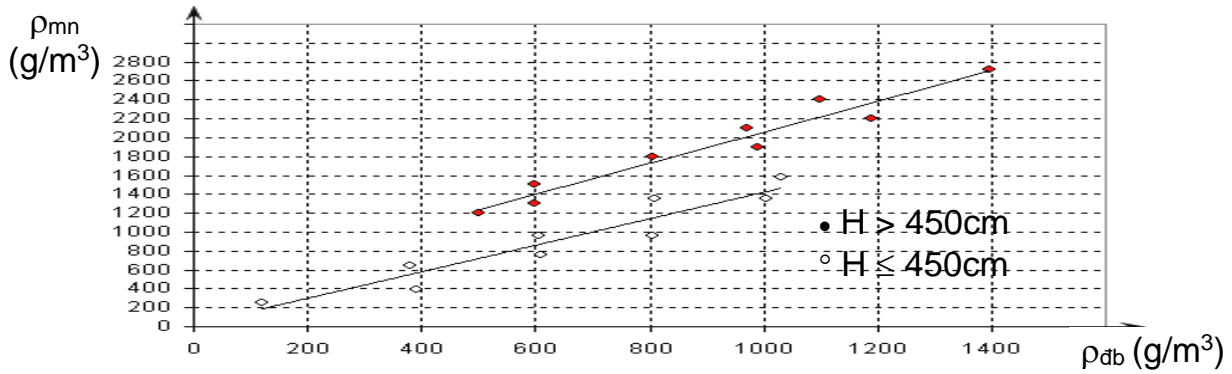
Hình D.2 - Tương quan \rho_{mn} = f(\rho_{db}) có phần mực nước cao tách khỏi mực nước thấp
