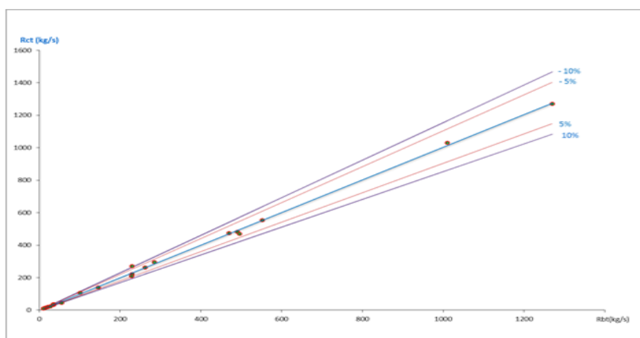
Hình 2 - Tương quan lưu lượng chất lơ lửng đo chi tiết và đo bình thường
