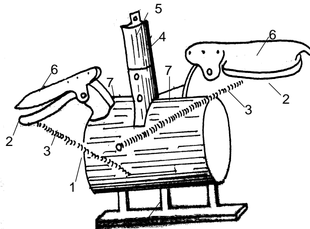
Hình A.4 - Thiết bị kiểu ngang
