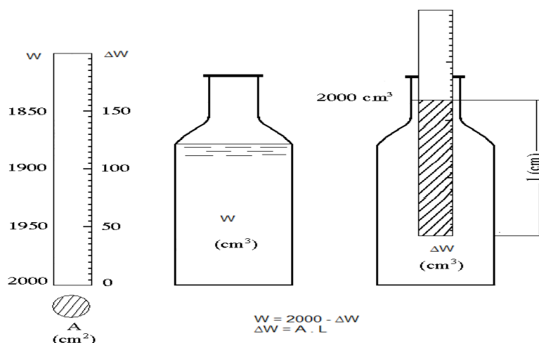
Hình 3 - Xác định thể tích mẫu nước
