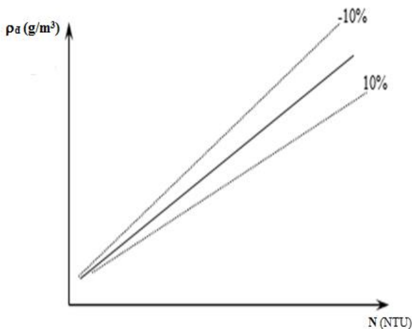
Hình 1- Tương quan giữa hàm lượng chất lơ lửng với độ đục thực đo
