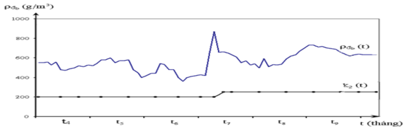
Hình D.5 - Biểu đồ đường quá trình hàm lượng chất lơ lửng đại biểu và sự thay đổi của hệ số k_2 theo thời gian
