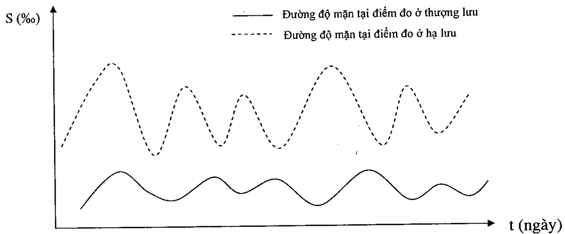
Hình 3: Đường quan hệ độ mặn giữa 2 điểm đo
